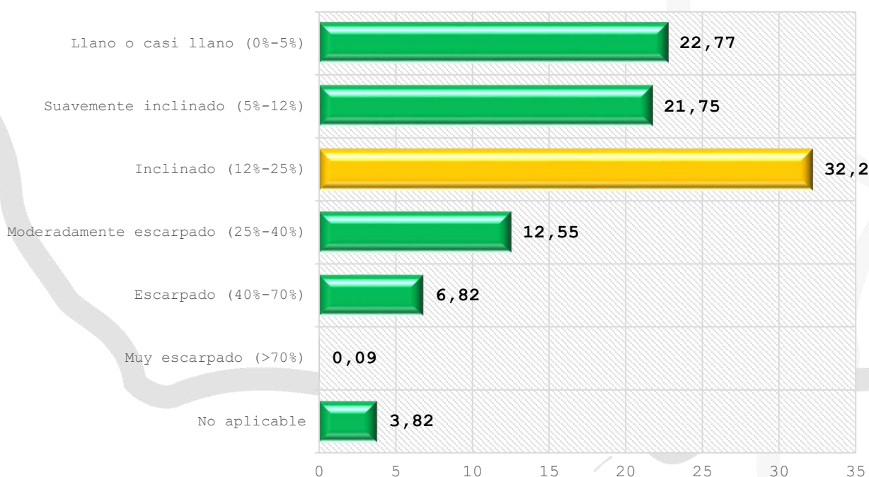
Ilustración 15: Pendientes
