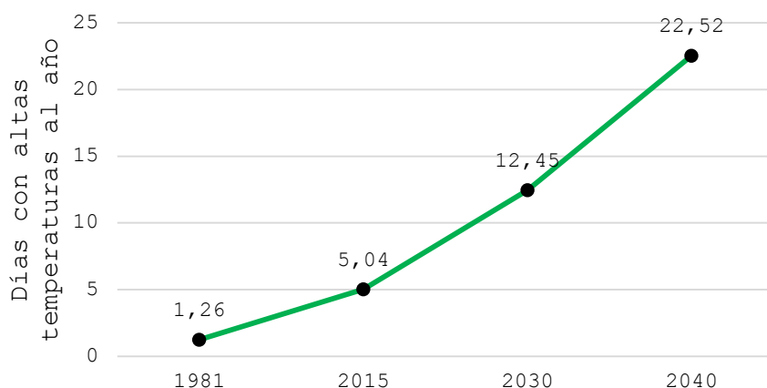
Ilustración 29: Altas Temperaturas-RCP 8.5
