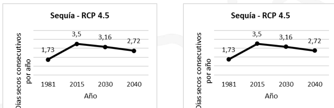
Ilustración 25: Sequía-RCP 4.5 / Sequía-RCP 8.5
