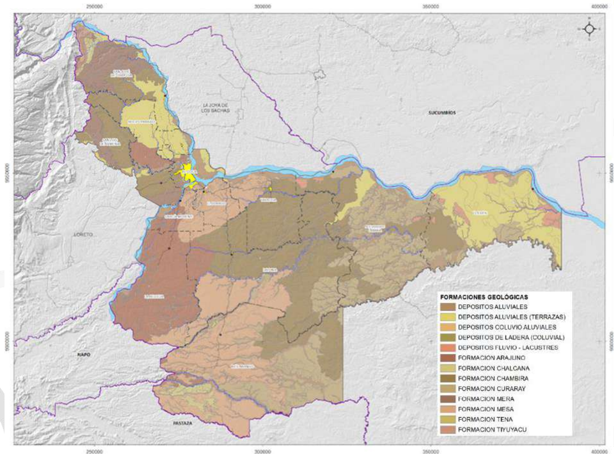
Mapa 3: Geología
